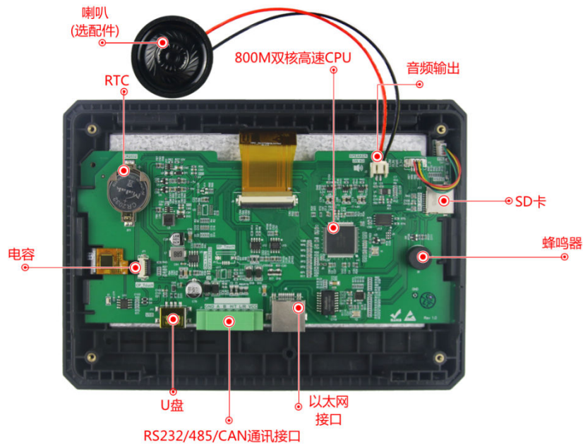
图 1-2 硬件配置图
